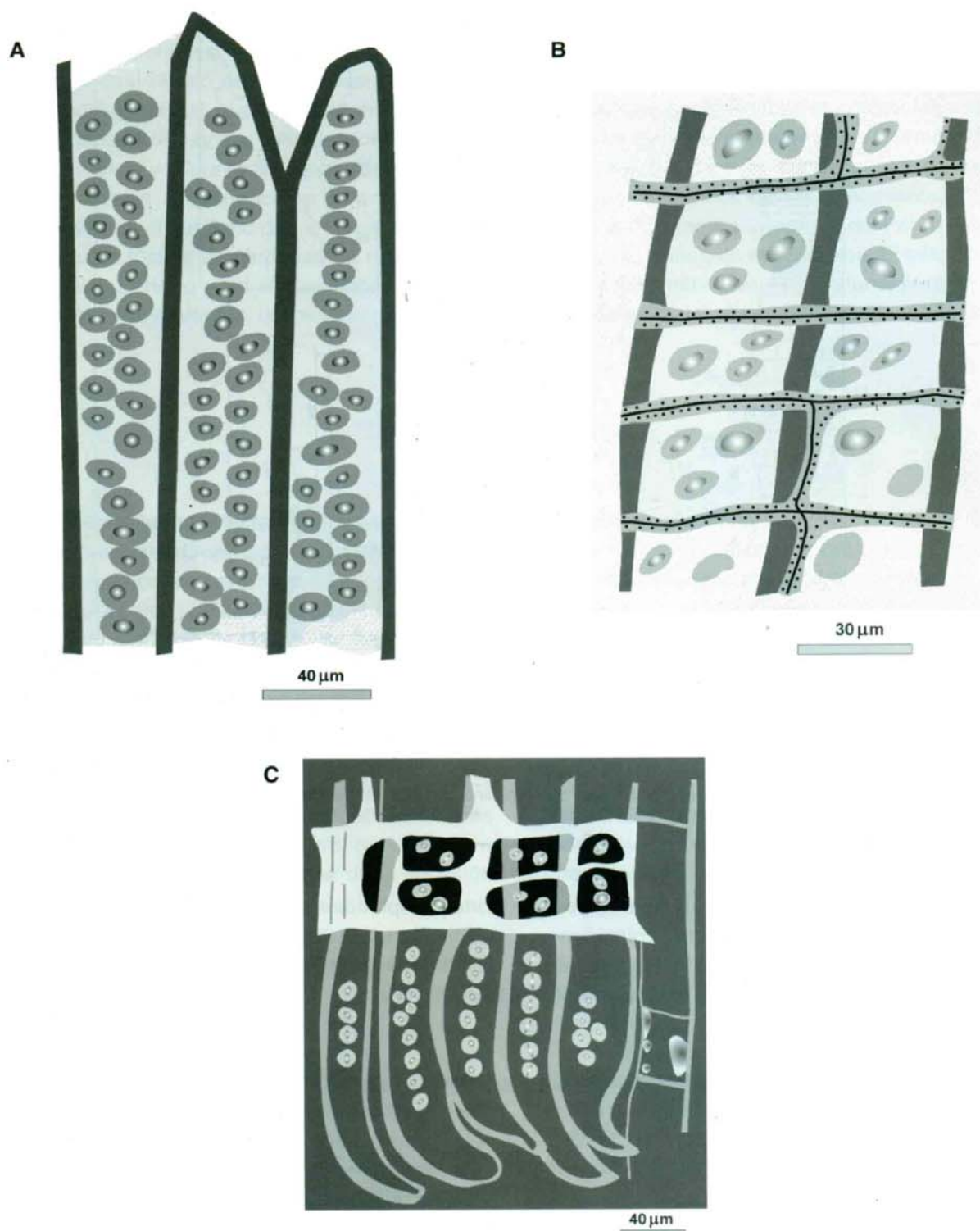
FIG. texto 2. Agathoxylon liguaensis sp. nov. A - traqueidas; B - campos de cruce con 1 a 3 puntuaciones. Baieroxylon chilense sp. nov.; C - vista radial que muestra las traqueidas torcidas y los campos de cruce.
